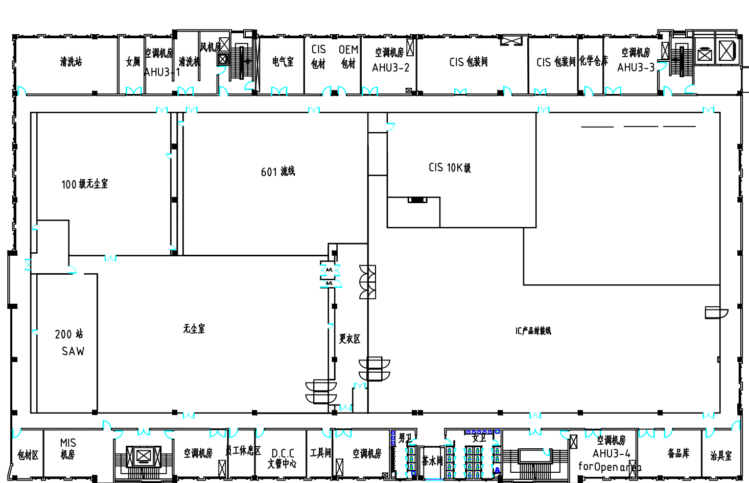
图4-3 车间平面布置图 (三层)
